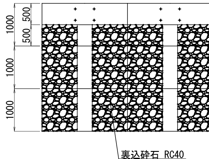
裏込砕石詳細図(背面図) S=1:50
