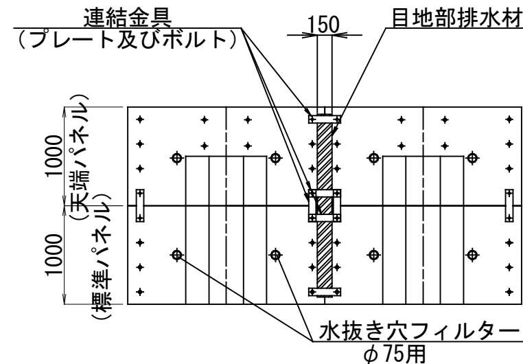
連結金具・取付詳細図 S=1:50
