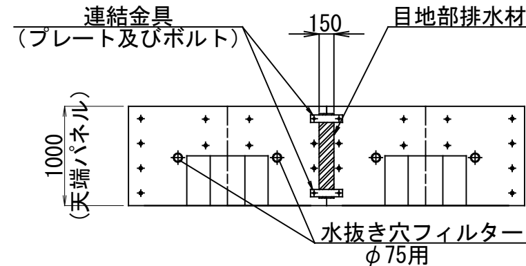
連結金具・取付詳細図 S=1:50
