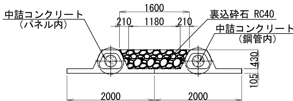
中詰コンクリート・裏込碎石詳細図 S=1:50
