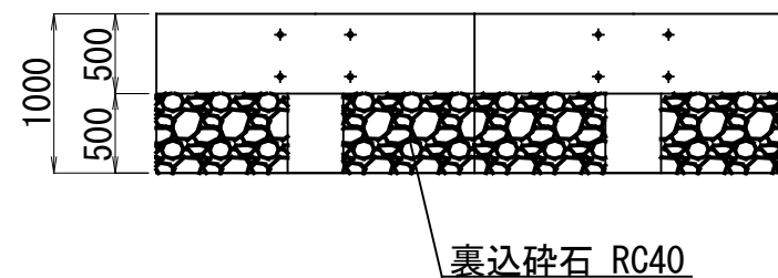
裏込碎石詳細図(背面図) S=1:50
