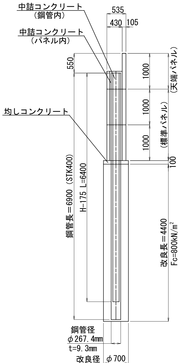
標準断面図 S=1:50 (柱状地盤改良体含む)
