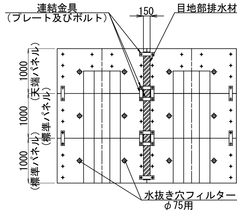
裏込砕石詳細図(背面図) S=1:50
