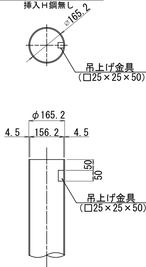
鋼管頭部詳細図 S=1:10 挿入H鋼無し
