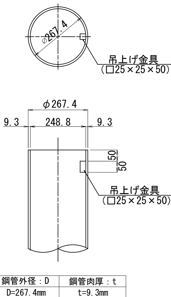
鋼管頭部詳細図 S=1:10 挿入H鋼無し
