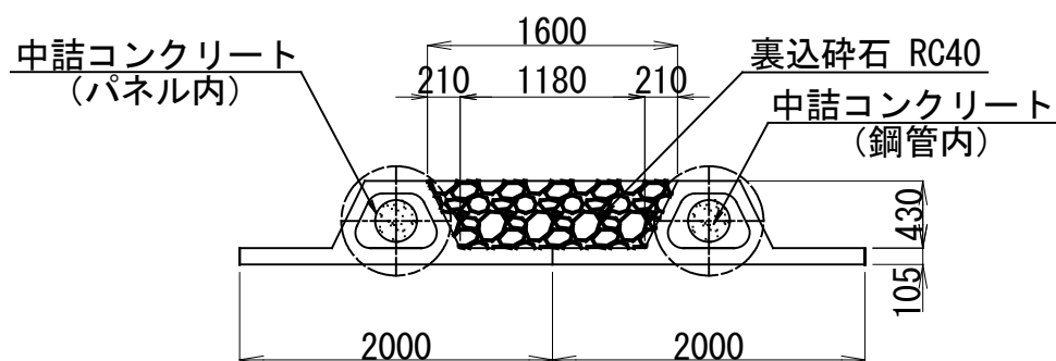
中詰コンクリート・裏込砕石詳細図 S=1:50
