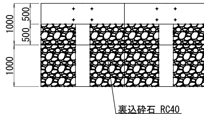
裏込砕石詳細図(背面図) S=1:50
