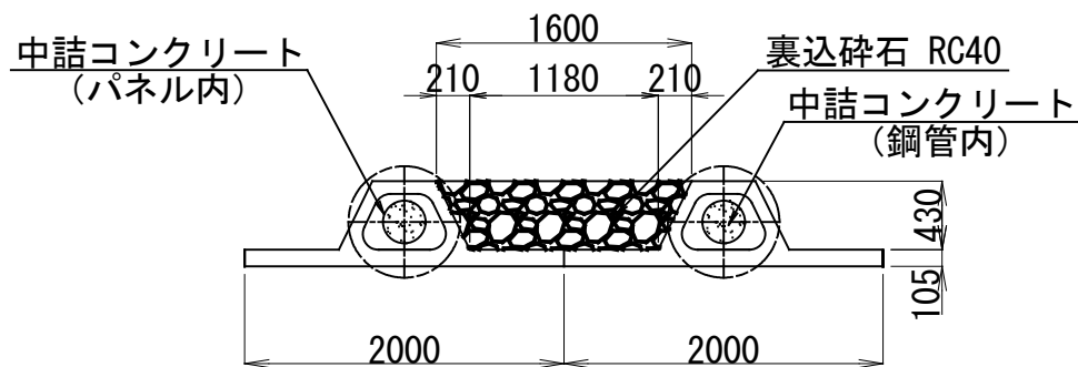
中詰コンクリート・裏込砕石詳細図 S=1:50
