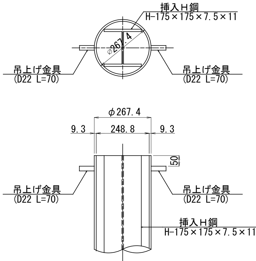
鋼管頭部詳細図 S=1:10 挿入H鋼: H-175
